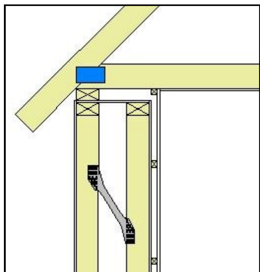
Detail připojení střechy ke stěně
