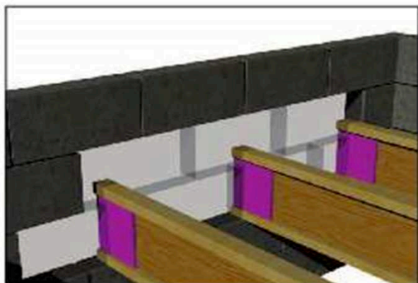
I-nosník: podporový detail
